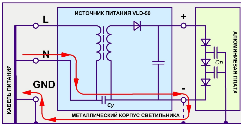
Рисунок 3. Схема шунтирования светодиодов
